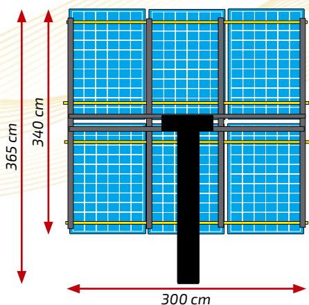
Dwuosiowy stojak obrotowy DSO-6PV – wymiary
